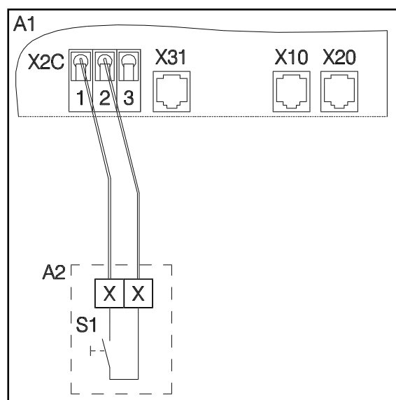
9 sz. ábra.: Az impulzus nyomógomb csatlakozása
