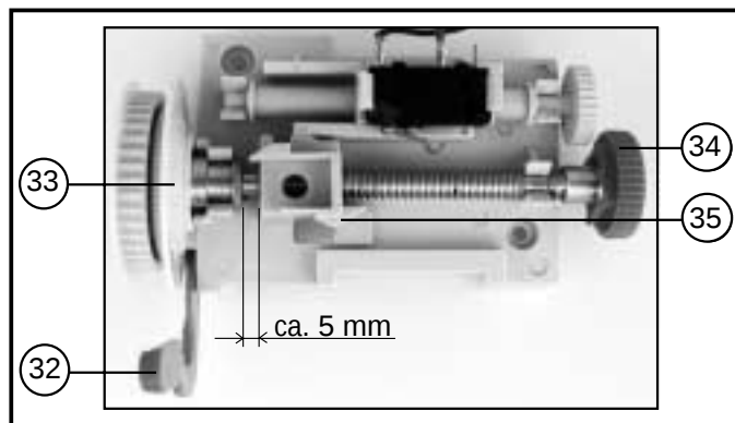
6. sz. ábra: Referenciapont beállítása (KAPU ZÁRVA)
