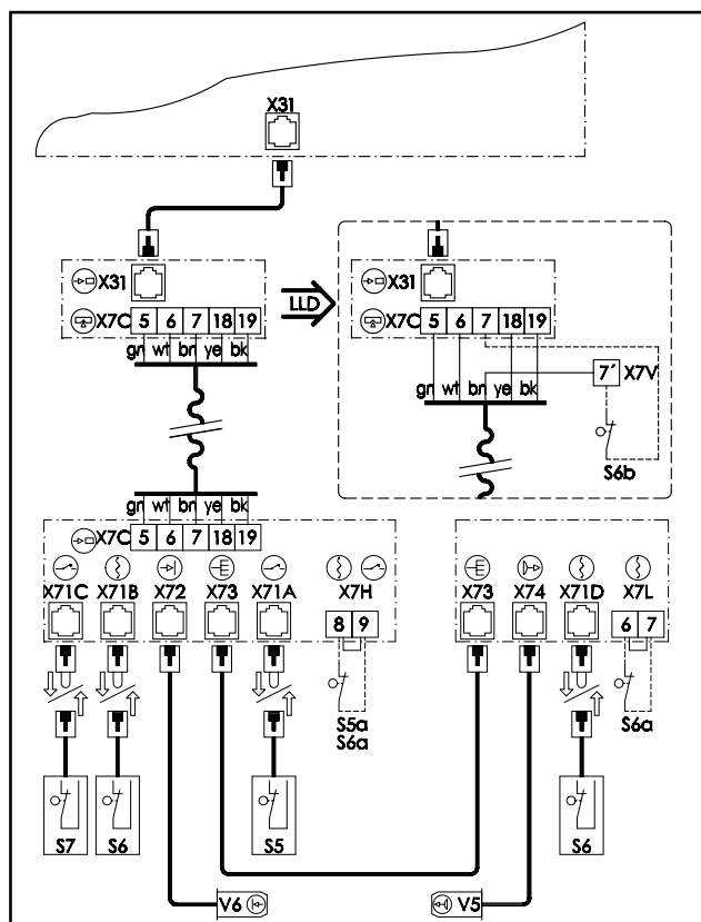
8. sz. ábra: Záróél-biztosítás kapcsolási rajza
