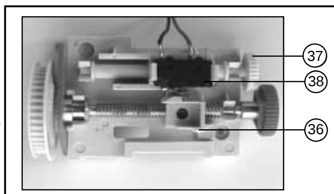
7. sz. ábra: A referenciapont beállítása
