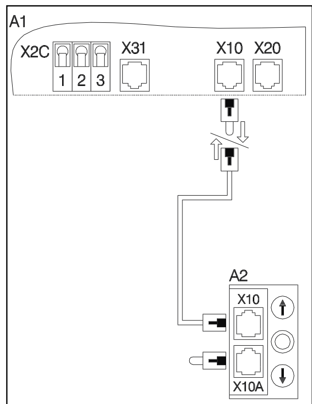
4.sz. ábra: a fóliabillentyűzet csatlakoztatása
